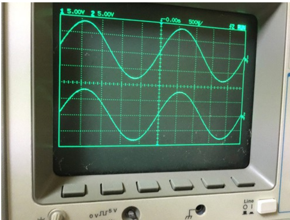
MM-MC時 3Ω時の波形 0.5V入力時 (1kHz) 36倍 16V出力
