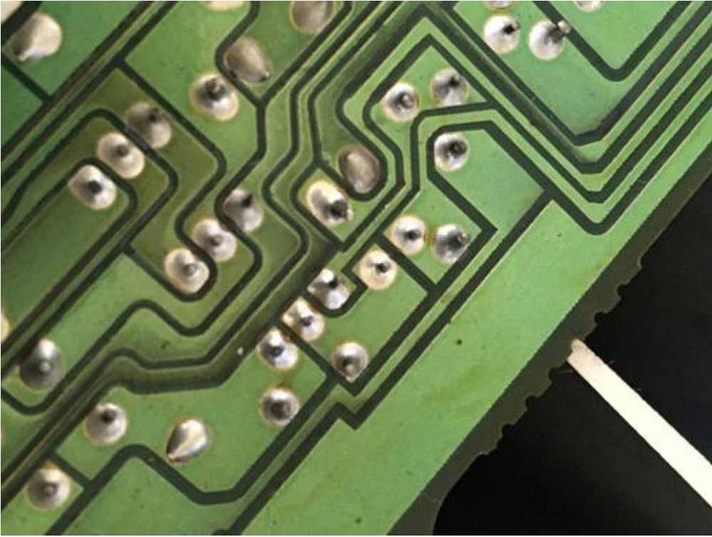
パワーアンプ基盤のはんだ異常箇所
