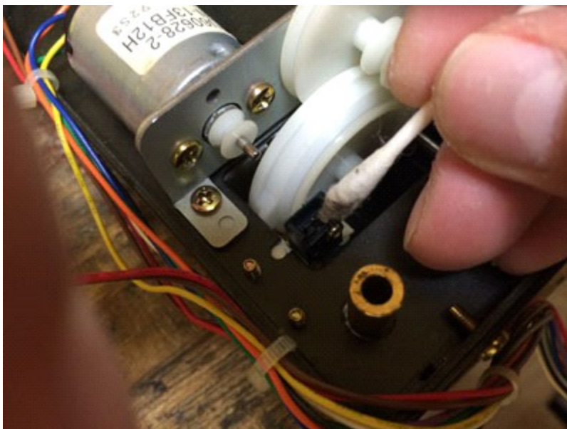
リフトアップ部分の分解、清掃
