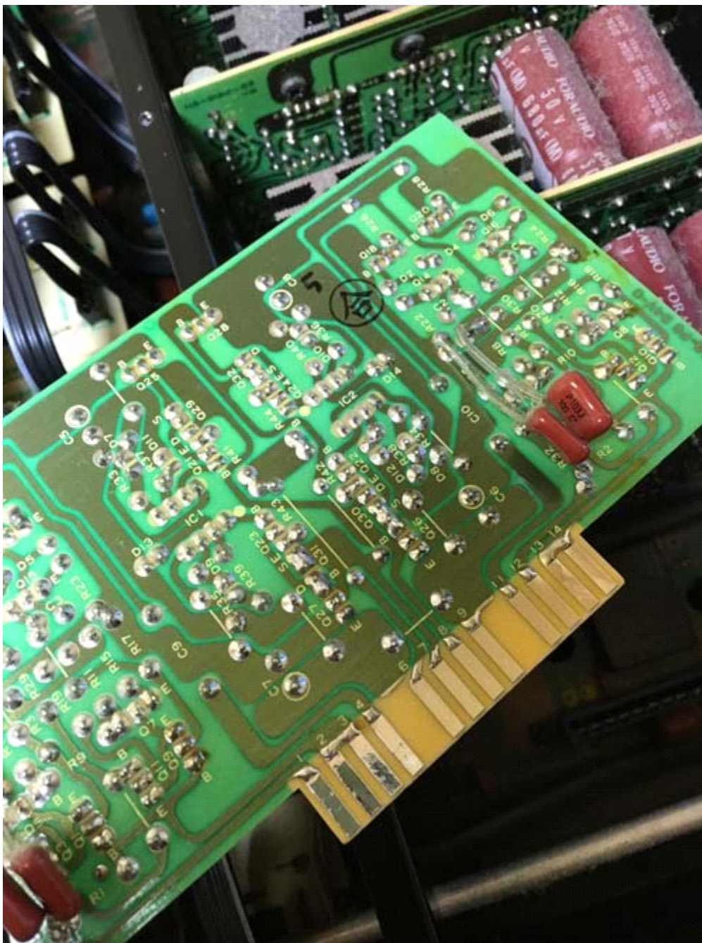
コネクタ部分のはんだ修正
