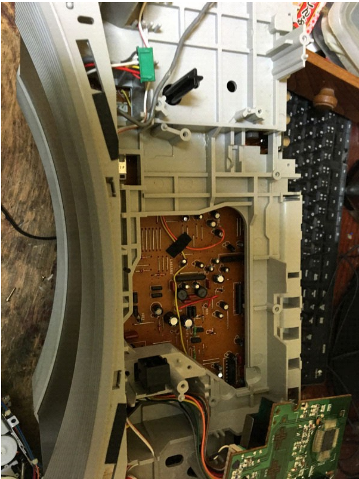
メカ分解開始、劣化グリースが黄ばんでいる
