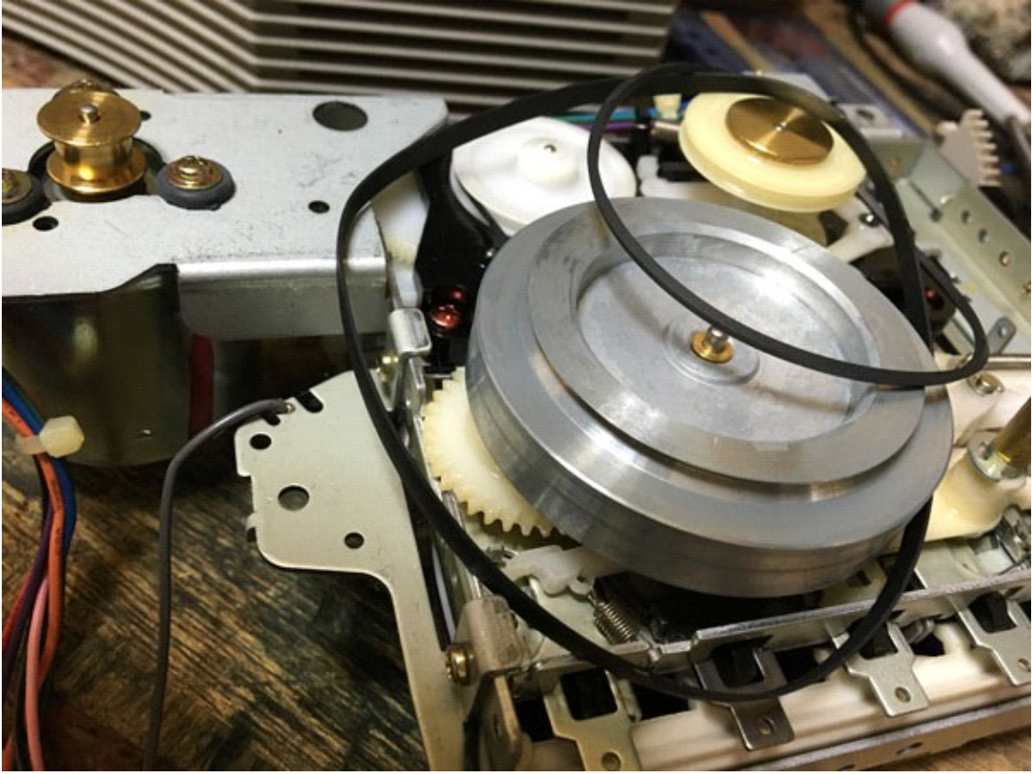
清掃後の状況
