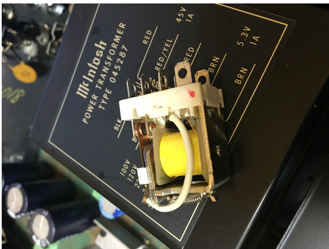
アウトプットリレーの接点清掃
