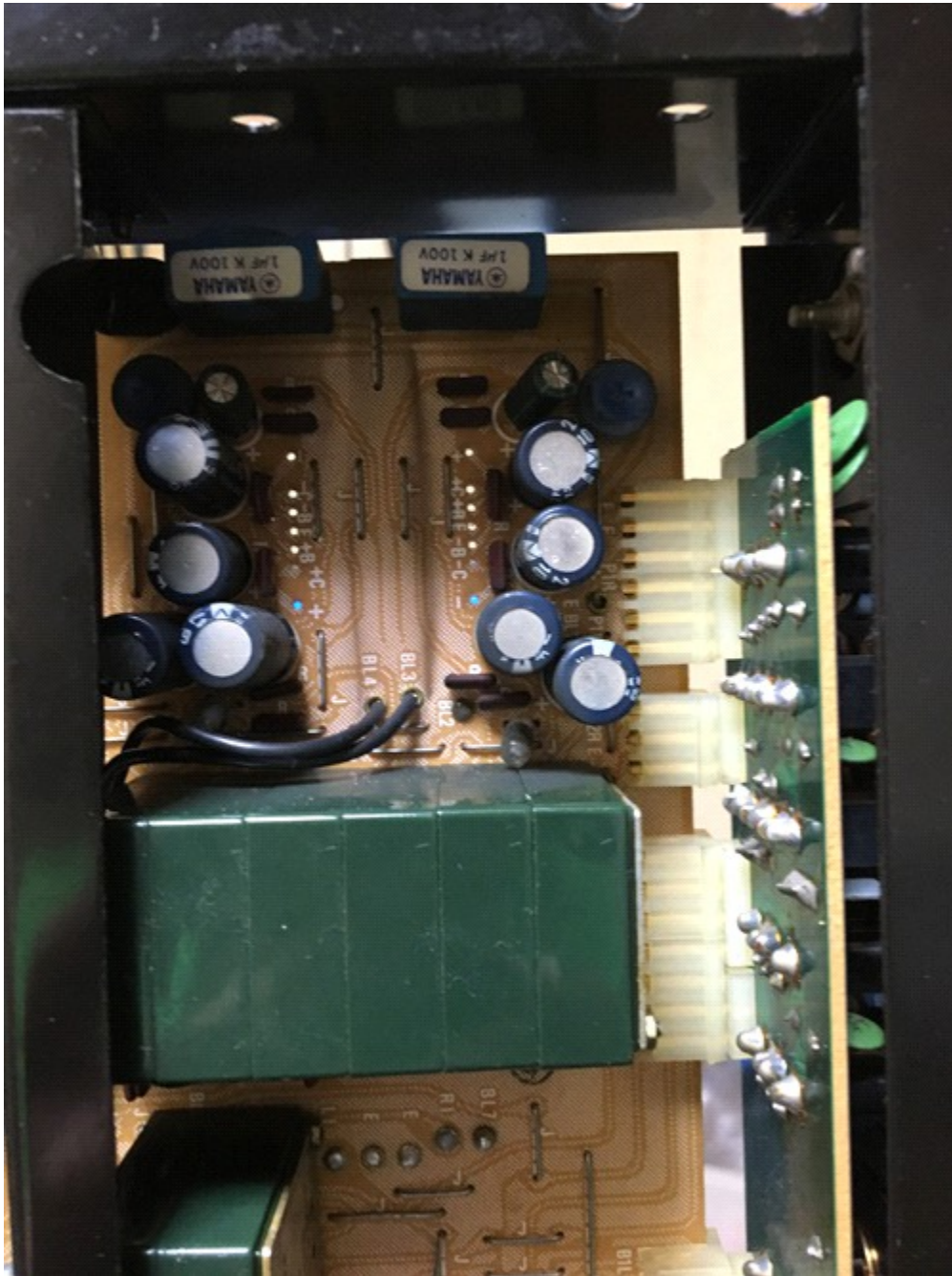
フォノイコライザー回路取り外し修理
