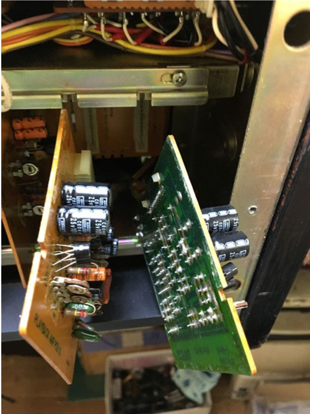
断線箇所の回路
