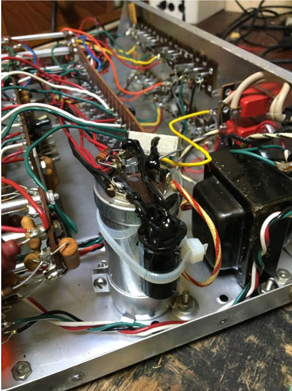
電源コンデンサー追加
