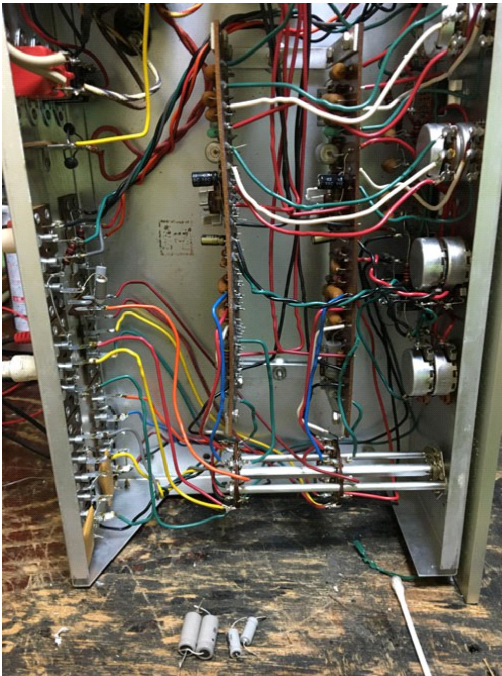
トーン回路、劣化コンデンサー交換
