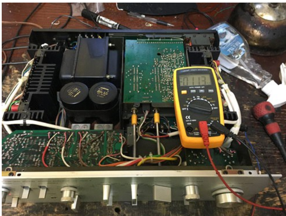
BIASやDCオフセットの調整
