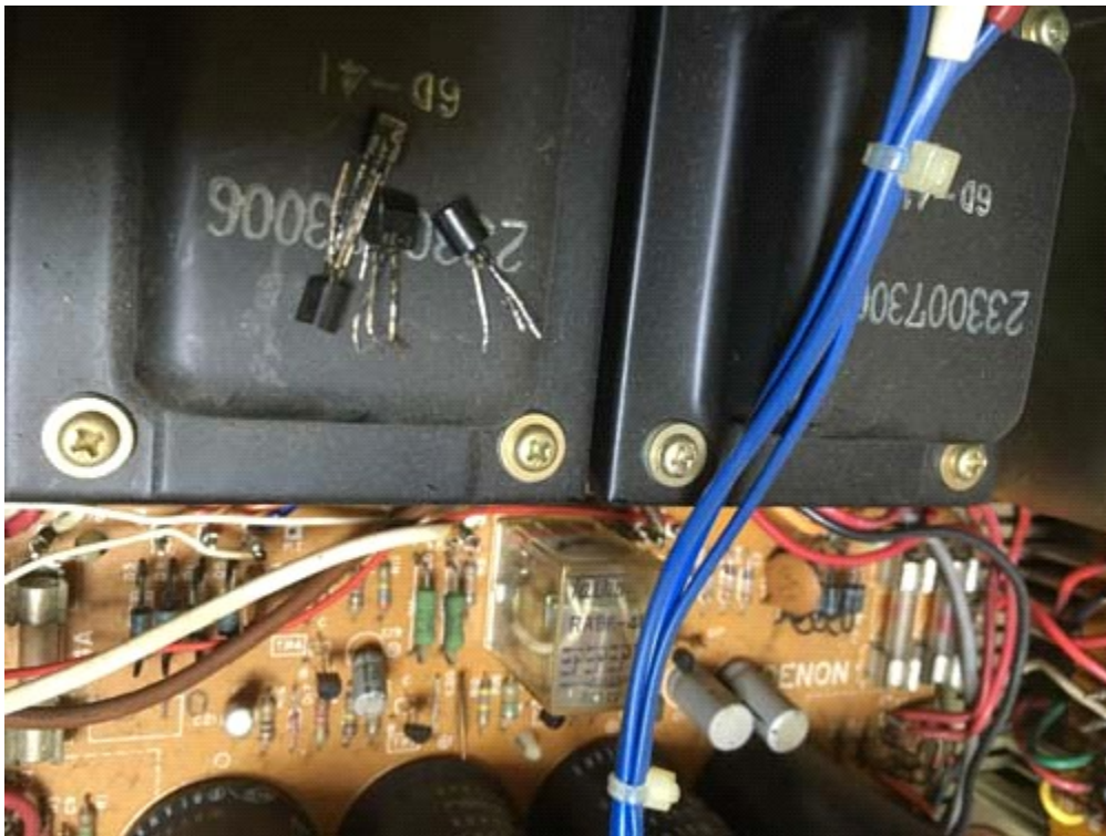
劣化トランジスター（プロテクト回路） またBIASの調整を済ませる
